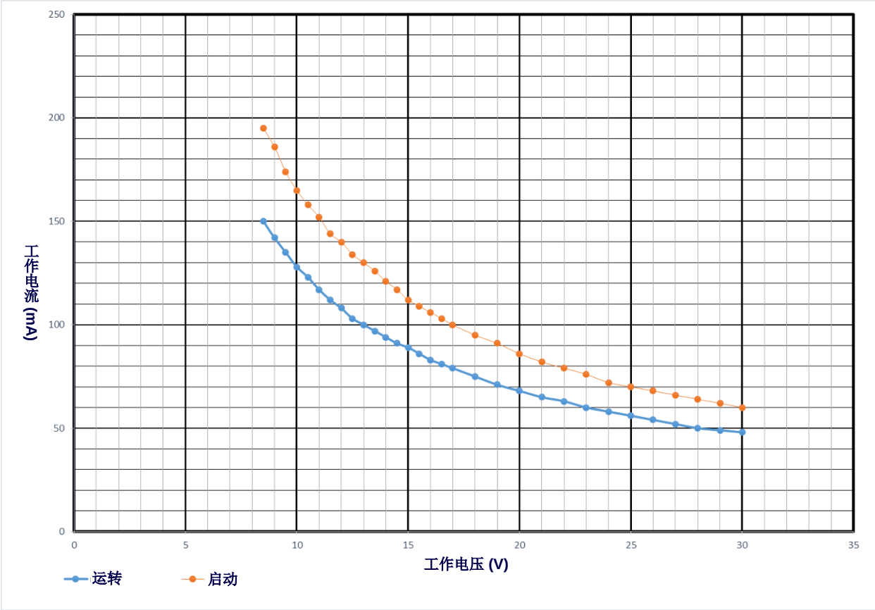
CS141 产品系列之功率消耗曲线图:
