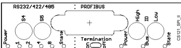
Abb. 2: Frontblende: Drehschalter, Leuchtanzeigen und Terminierung PB
