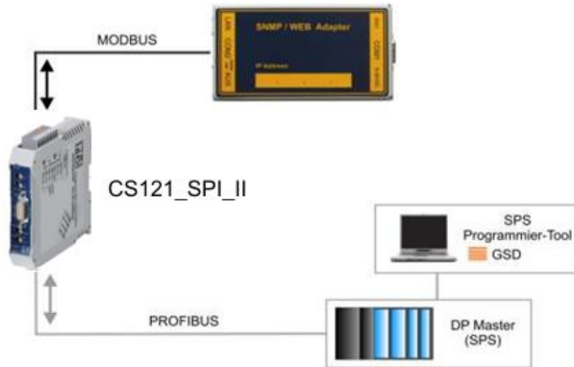
Abb. 7: Anschlussprinzip des CS121/BACS_SPI_II
