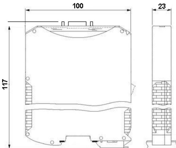
Abb. 6: Maßzeichnung CS121/BACS_SPI_II
