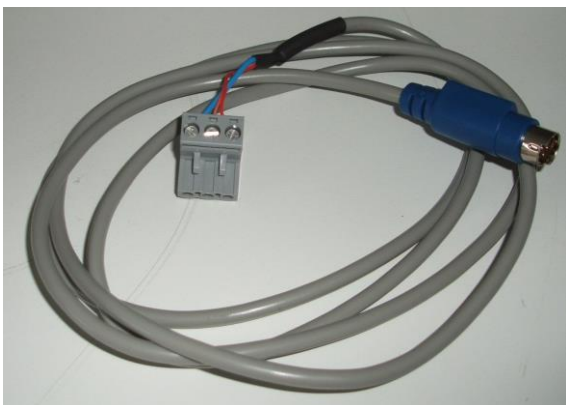
Abb. 4: Verbindungskabel CS121/CS141 COM 2 zu CS121/BACS_SPI_II
