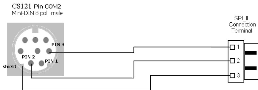
Abb. 3: PIN-Belegung Verbindungskabel CS121 / CS141 COM 2 zu CS121/BACS_SPI_II
