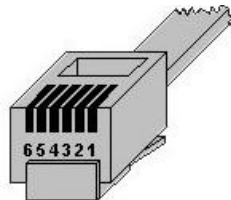
PIN-Belegung RJ12-Stecker
